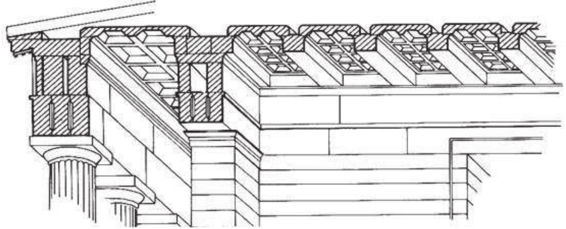
La cubierta del templo griego.
