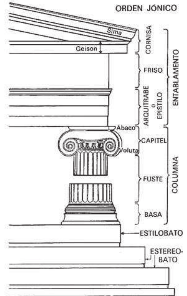
La columna jónica.
