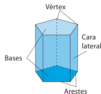
Prisma recte
