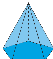
Piràmide pentagonal
