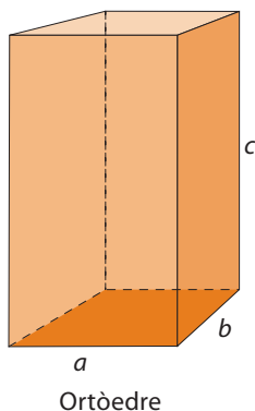
Ortòedre
