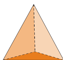
Piràmide triangular
