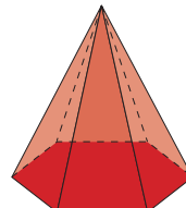
Piràmide hexagonal
