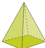
Piràmide quadrangular
